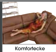
Relaxfunktion
